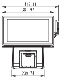
Printer Stand
